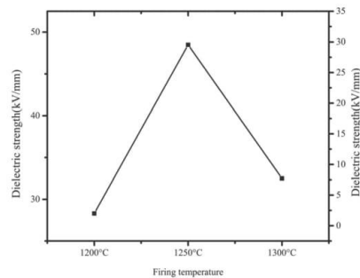
Fig. 4. Variation of dielectric strength of triaxial electrical porcelain sample versus the firing temperature Fig. 4. Triaxiális szigetelő porcelán dielektromos jellemzői az égetési hőmérséklet függvényében
